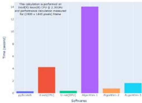
Şekil 6: Yöntemlerin saniye cinsinden yara tespiti hesaplama süreleri.
