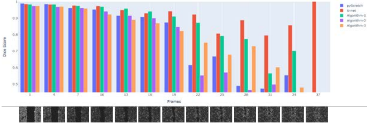
Şekil 4: Yöntemlerin her çerçeveye ait başarımları.
