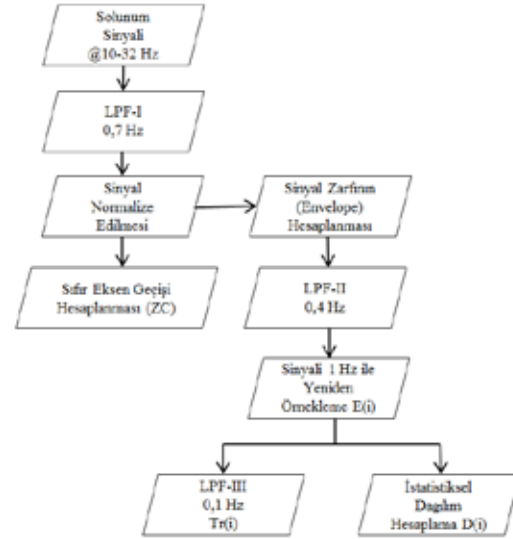
Şekil 1: Solunum Sinyalinden Apne Belirleme Algoritması 1. Bölüm
