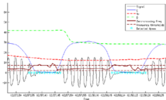
Şekil 4: Örnek Hasta Ayrıntılı Solunum Sinyali ve Apne Grafiği
