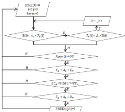
Şekil 2: Solunum Sinyalinden Apne Belirleme Algoritması 2. Bölüm
